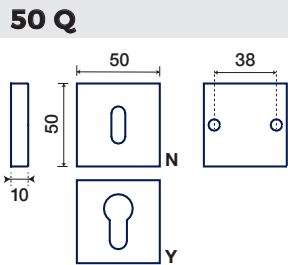
BOCCHETTA QUADRATA SQUARE ESCUTCHEON
